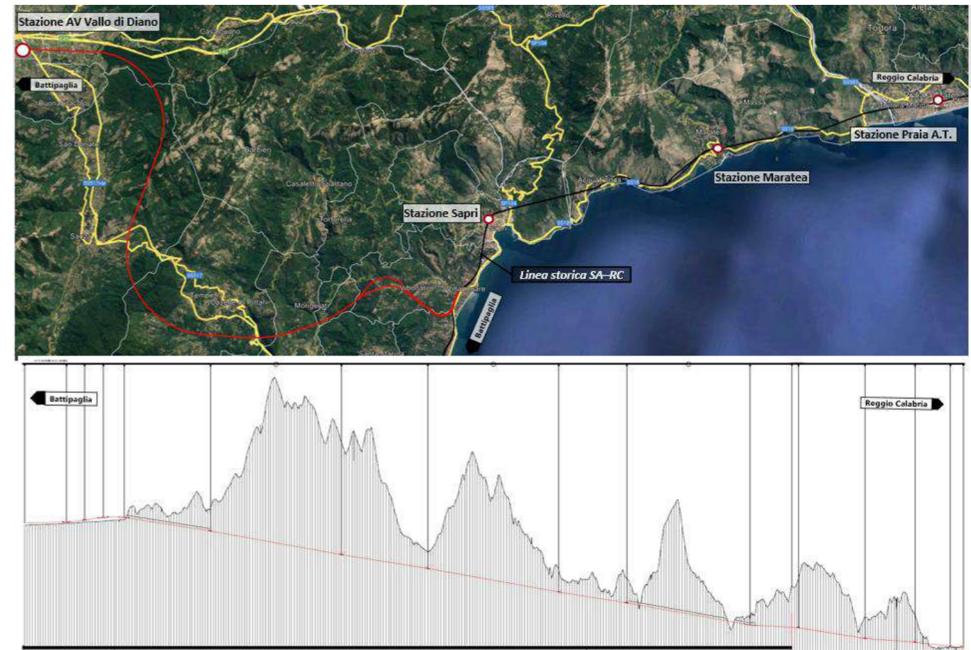
Figura 20 Profilo piano-altimetrico dell'alternativa di tracciato B
