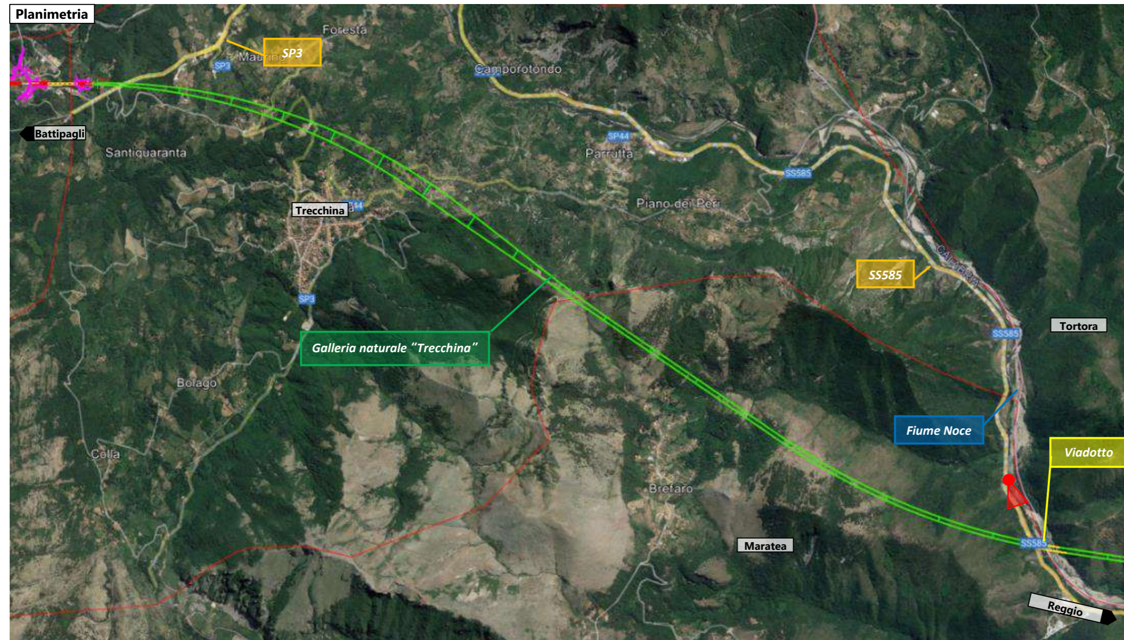
Figura 48 Vista planimetrica galleria naturale "Trecchina" e viadotto di scavalco fiume Noce
