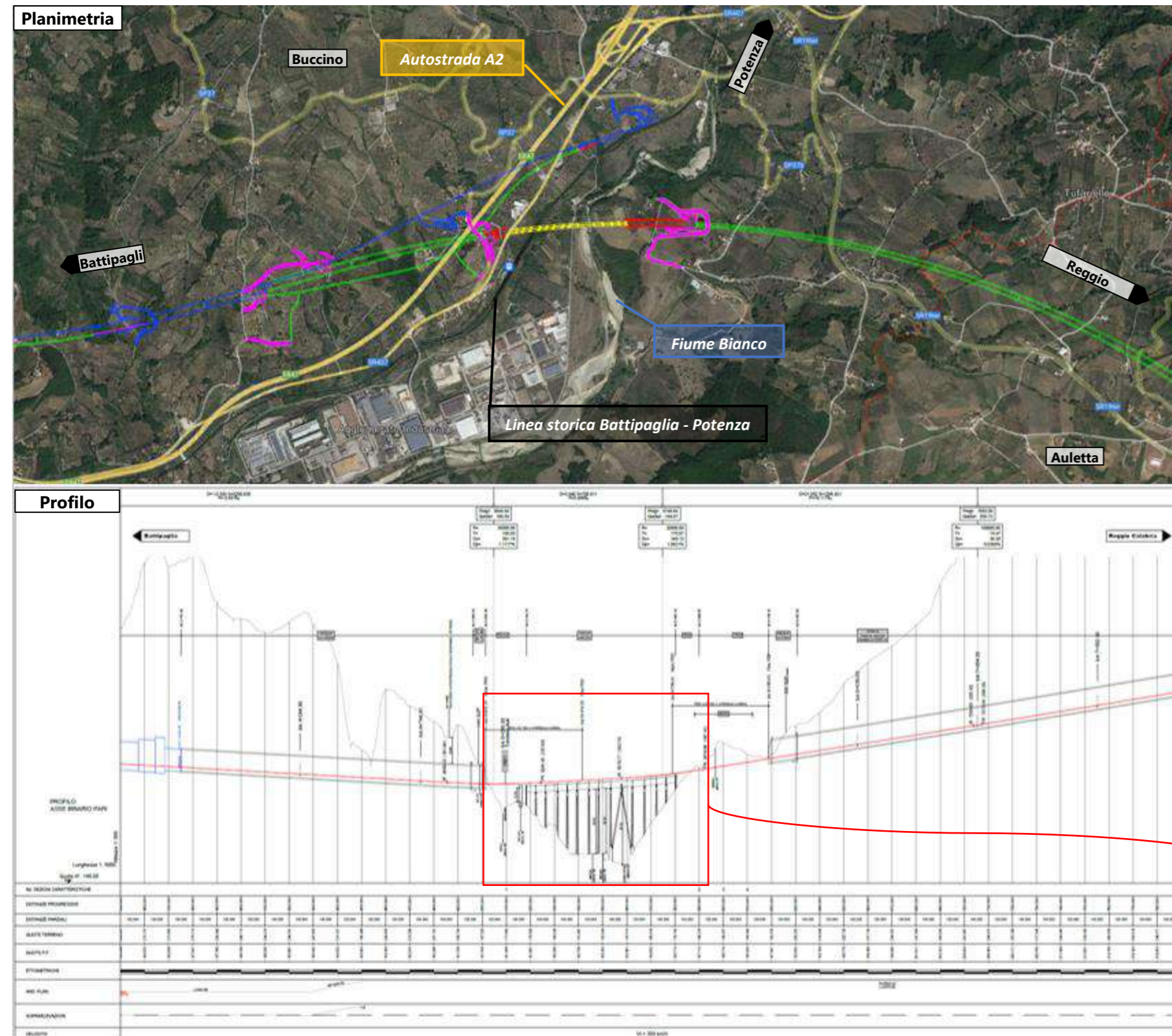
Figura 38 Plano profilo del tratto iniziale dell'intervento compreso tra il territorio del Comune di Buccino e di Auletta
