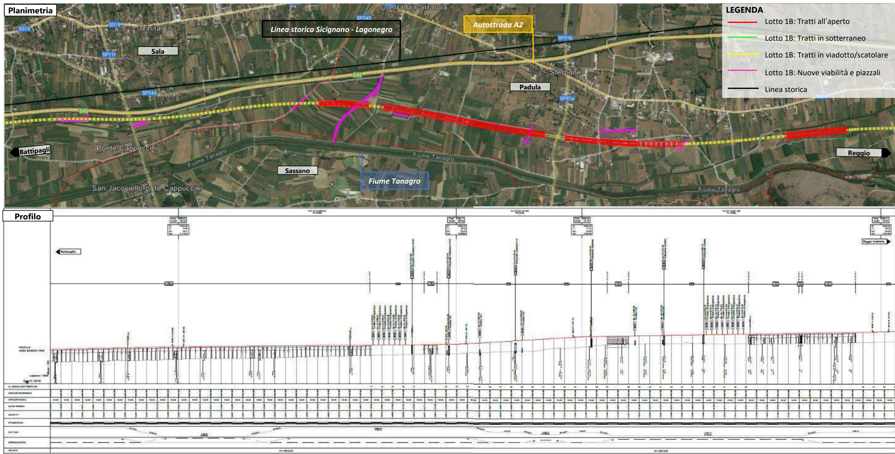
Figura 43 Sviluppo del tracciato all'interno del Vallo di Diano – Stralcio 4
