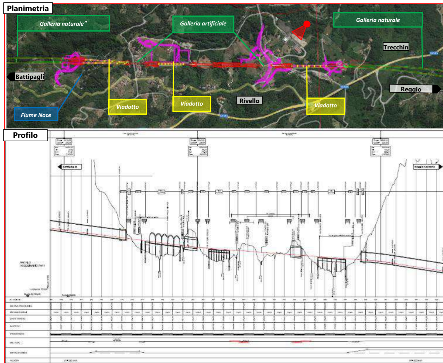
Figura 47 Piano profilo all'interno dei Comuni di Rivello e Trecchina
