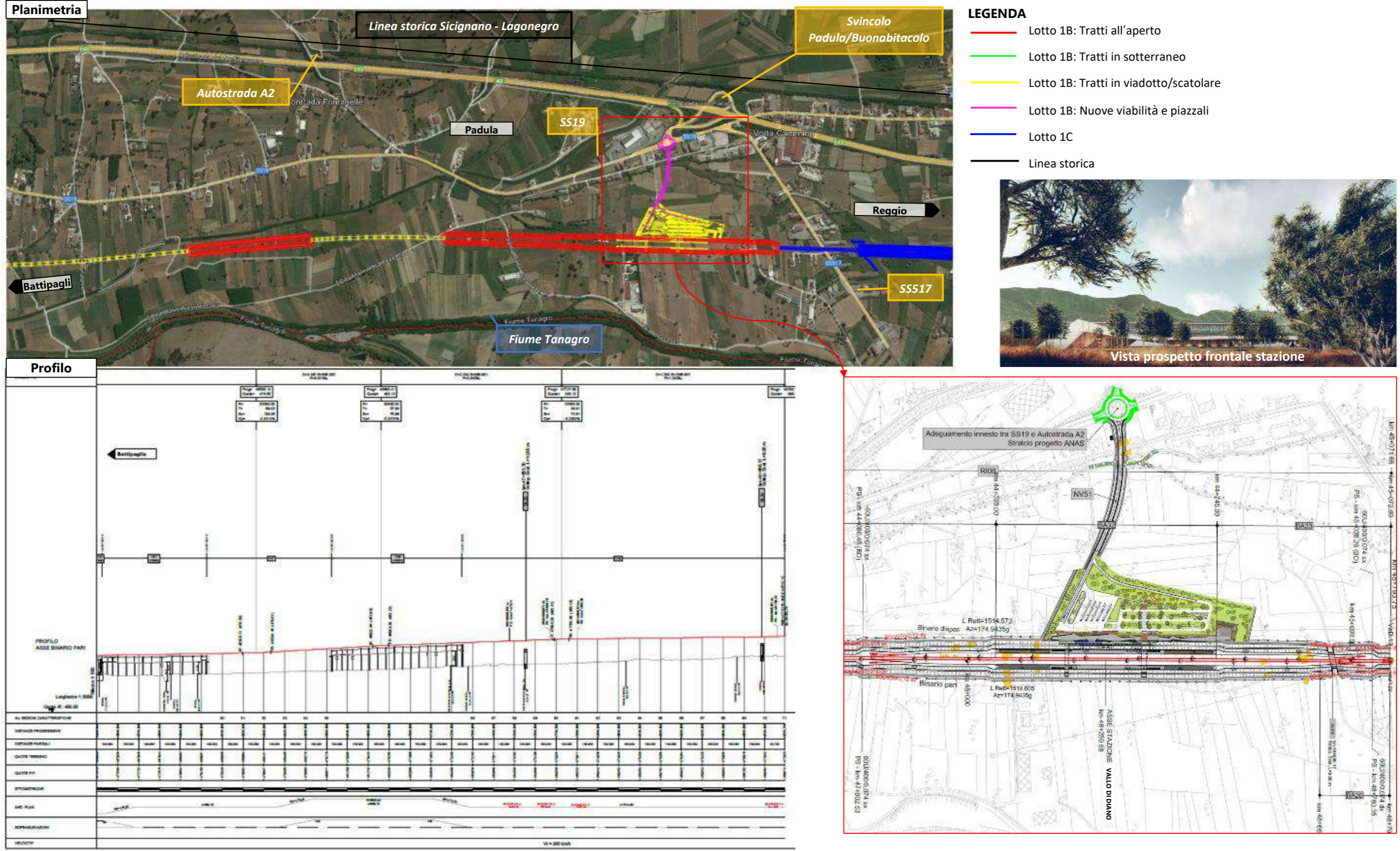
Figura 44 Sviluppo del tracciato all'interno del Vallo di Diano – Stralcio 5
