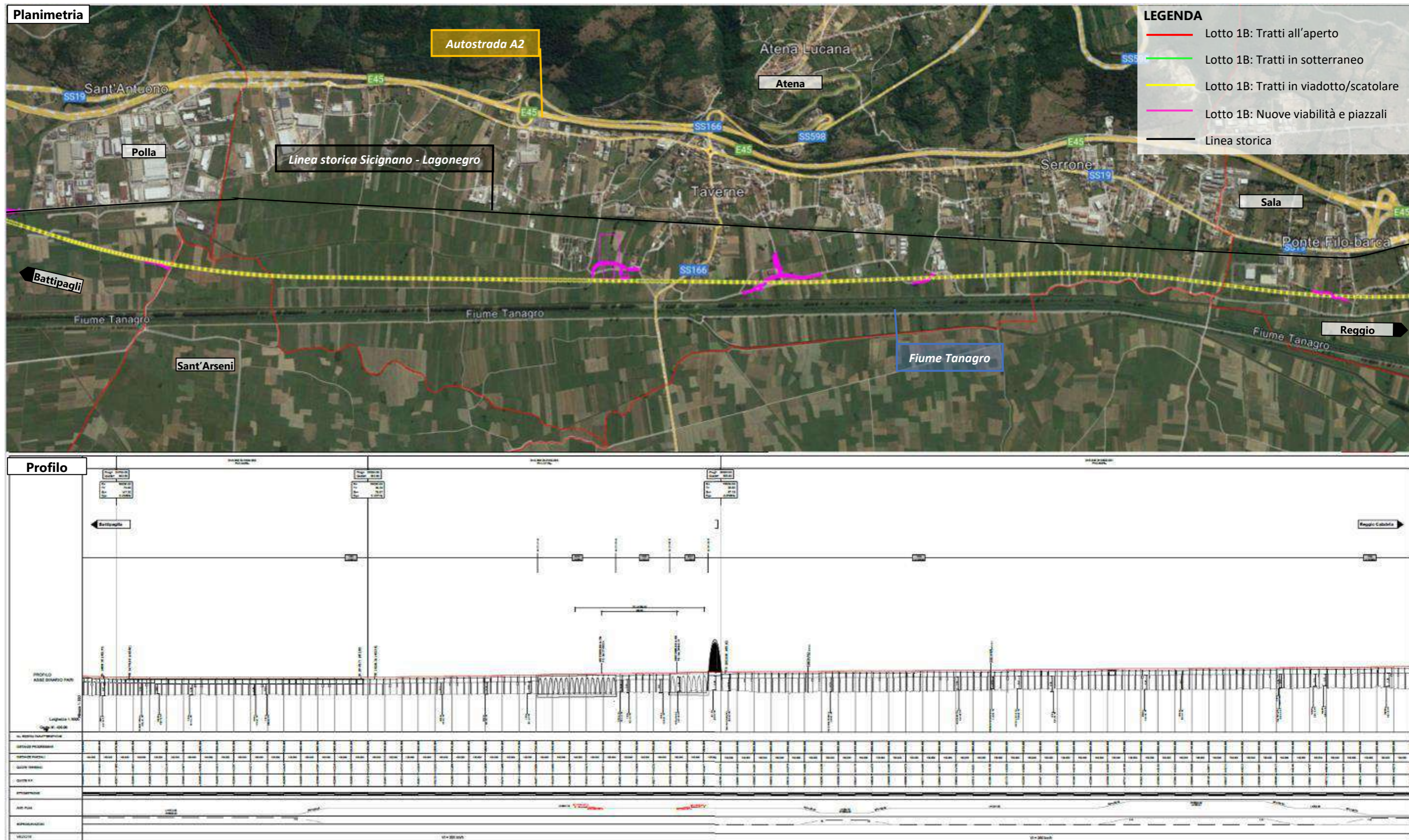
Figura 41 Sviluppo del tracciato all'interno del Vallo di Diano – Stralcio 2
